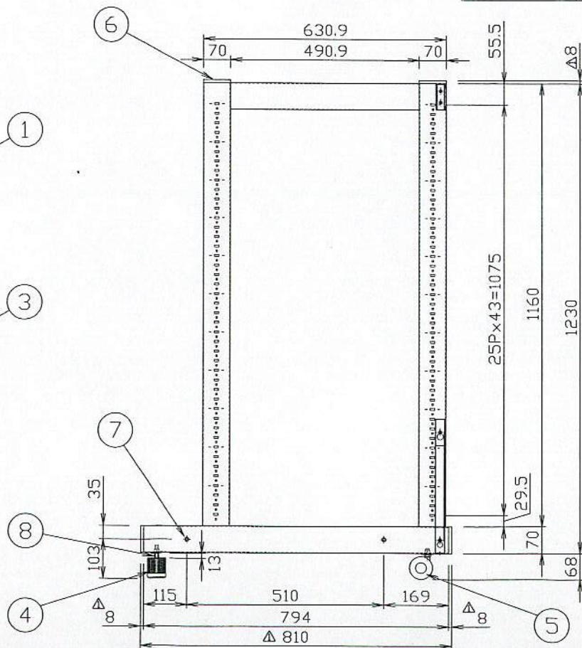
ア-ア矢視図
