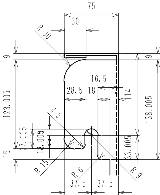
ア部詳細図 S=1/1
