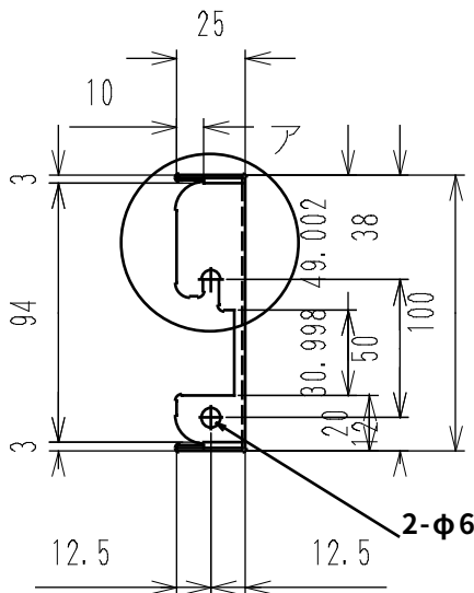
ア部詳細図 S=1/1
