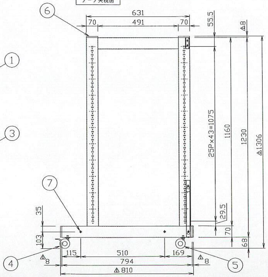
ア-ア矢視図
