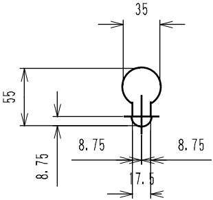
ア部拡大図 S=1/2
