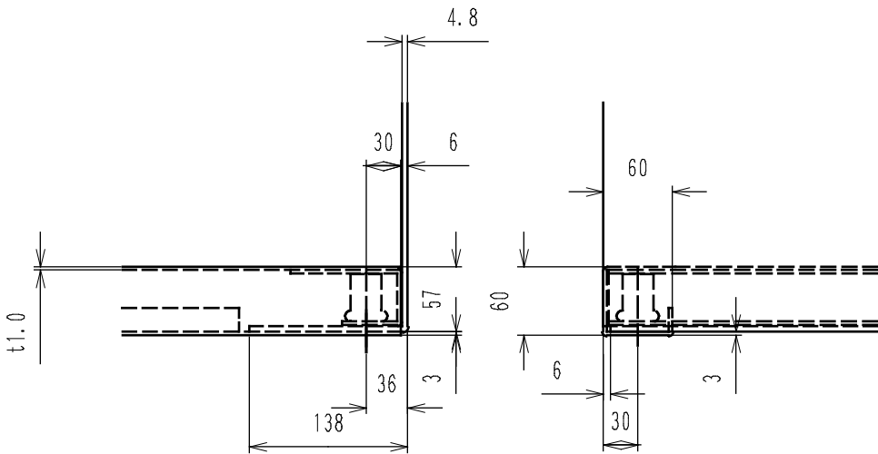
A部詳細図 S=1/2
