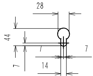
B部詳細図 S=1/3
