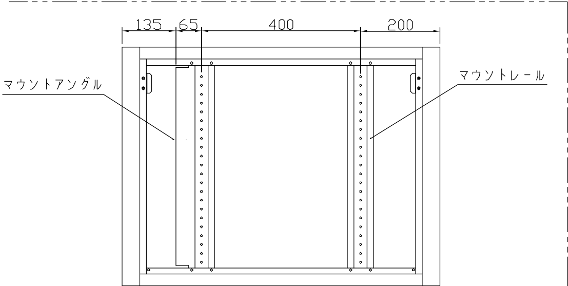
サイドパネルを外した状態
