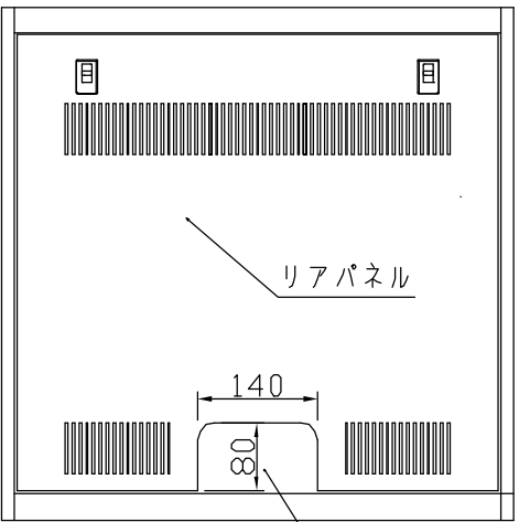
ケーブル通線孔
