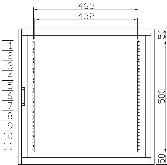
扉を外した状態
