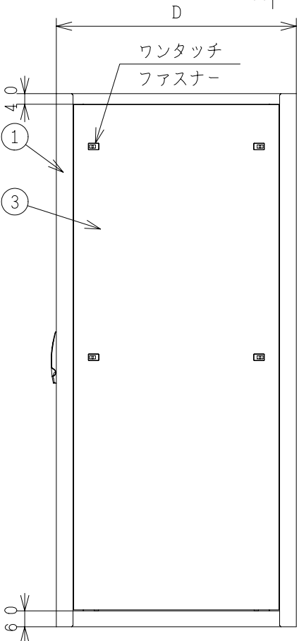
側面図
