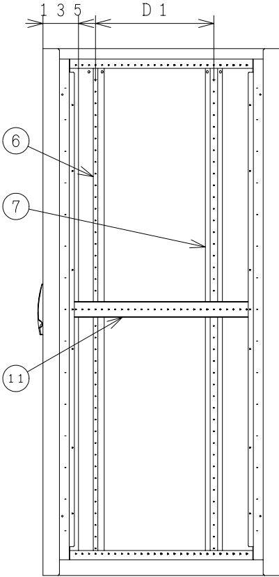
サイドパネルを外した状態
