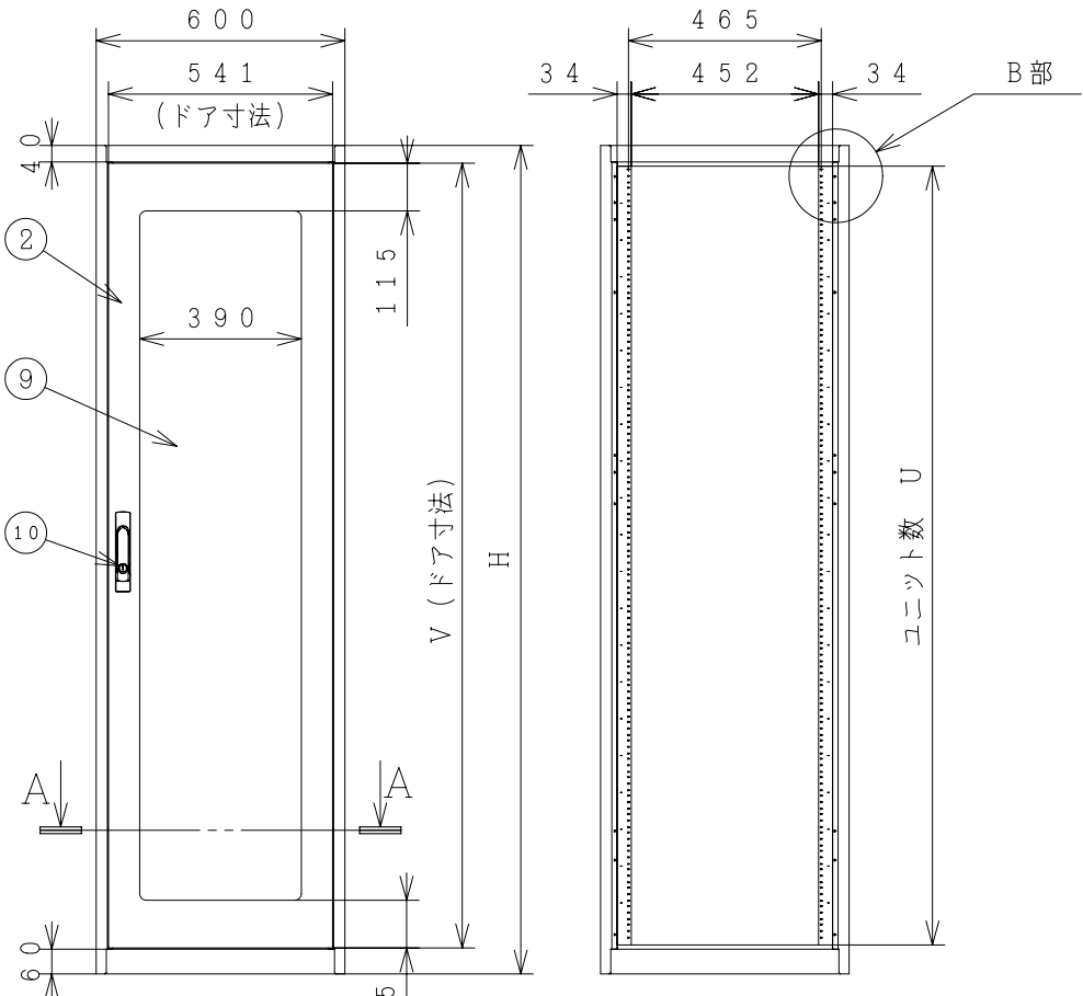
正面図
