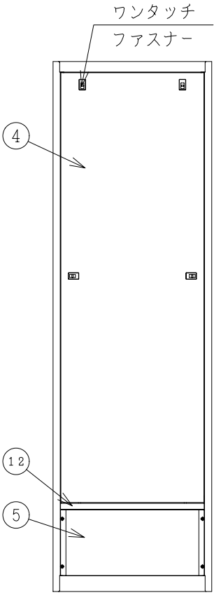
背面図
